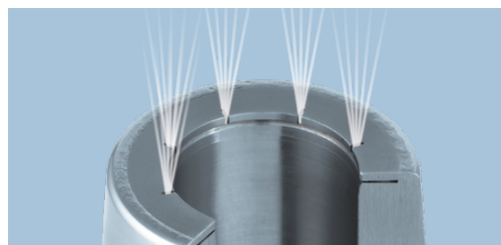
Optimierte Kühlmittelbohrung mit KSS-Austritt durch Schlitzte. Optimised coolant bores with coolant outlet through slots.
